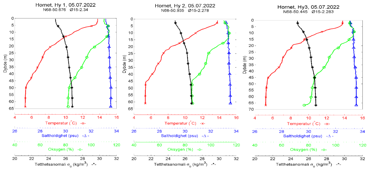
Figur 10. Vertikalprofiler for temperatur, saltholdighet, tetthet og oksygenivåer fra overflate til bunn på stasjonene Hy1, Hy2 og Hy3 den 05.07.2022.
